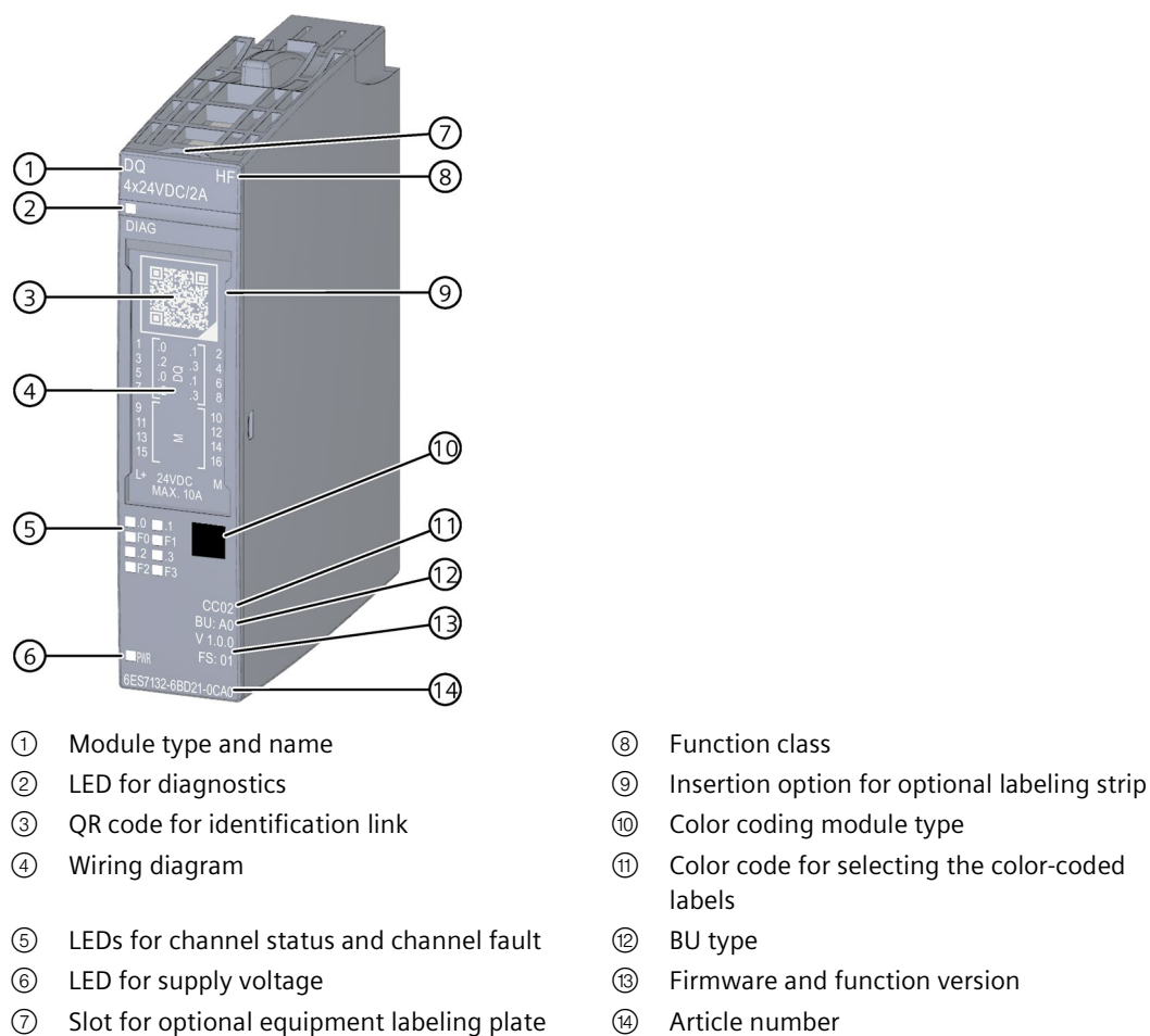
Figure 3-1 View of the module DQ 4x24VDC/2A HF
